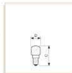
C D мм. мм. 57 25
