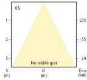
Диаграмма направленности светового пучка
