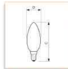
Размеры C D № макс. макс. 1 100 35
