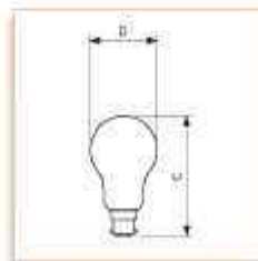
Размеры C D № макс. ном. 3 95,5 85
